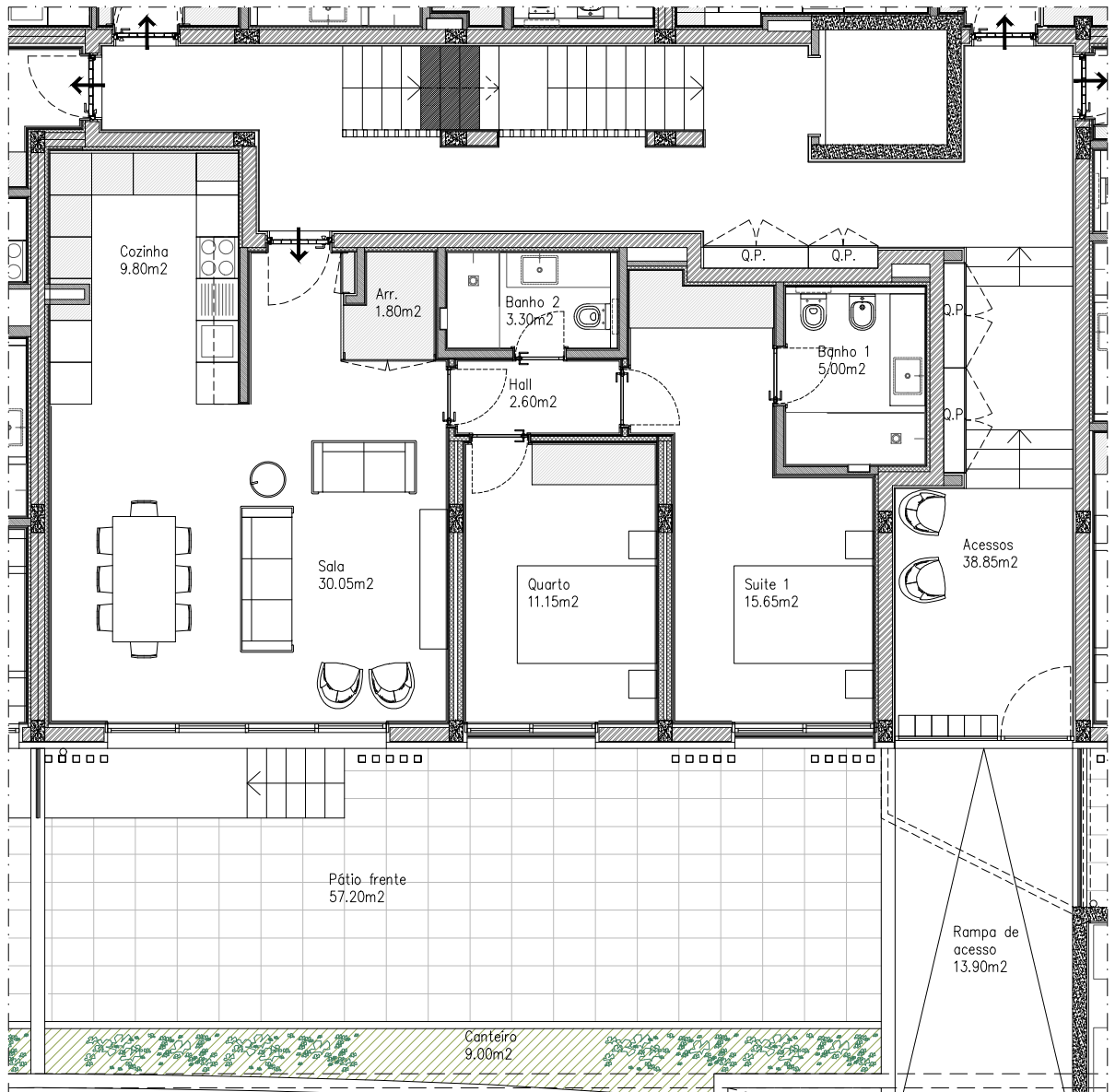
DESTAQUE PLANTA DA FRACÇÃO ESC. 1:100
