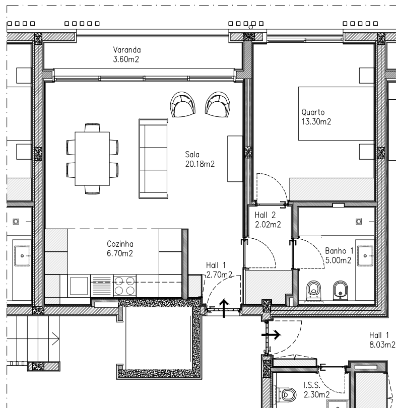
DESTAQUE PLANTA DA FRACÇÃO ESC. 1:100
