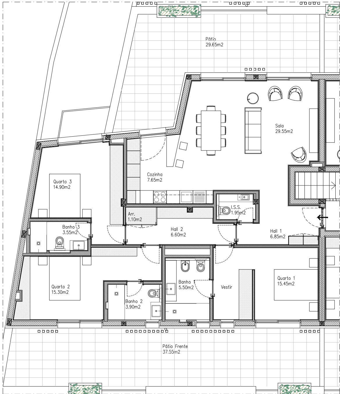
DESTAQUE PLANTA DA FRACÇÃO ESC. 1:100
